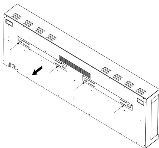
UNIQUE 180 PRO Muurbeugel geïllustreerd
