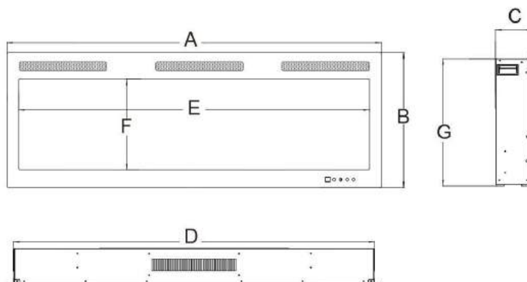
ROZMĚRY VÝROBKU
