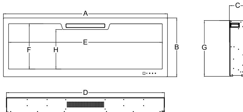
ROZMERY VÝROBKU
